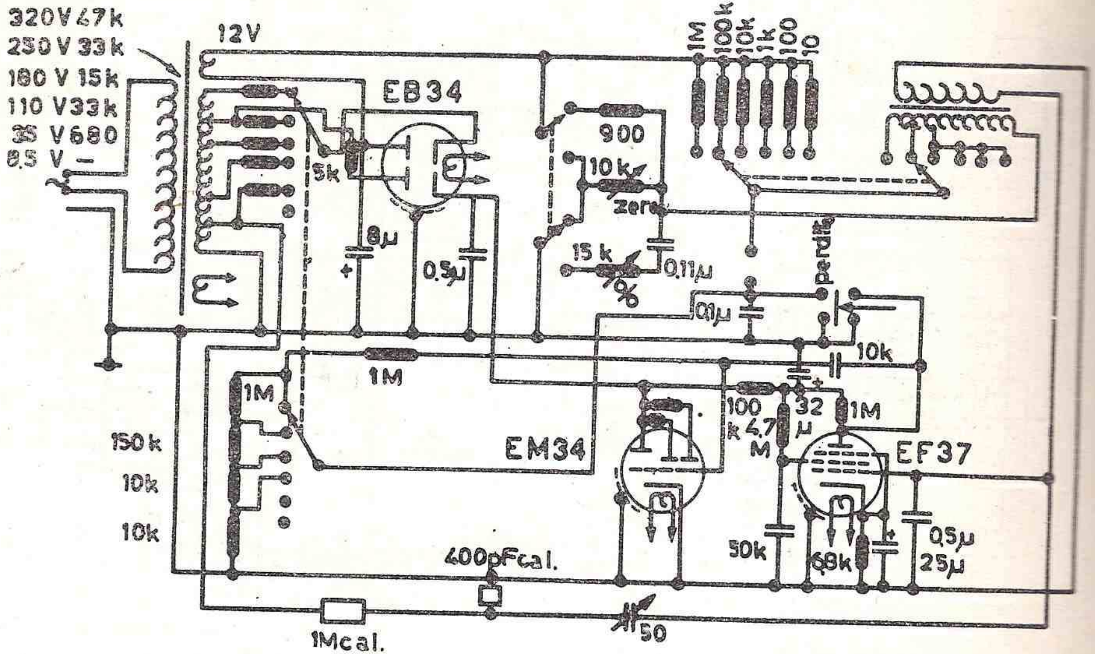
Fig. 74. - Ponte della British Physical Laboratories RS-700.
